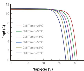
Wykres prąd-napięcie
